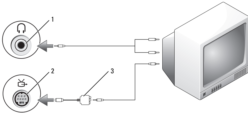
1 音效輸入連接器 2 分離式影像電視輸出連接器 3 合成式影像配接器
