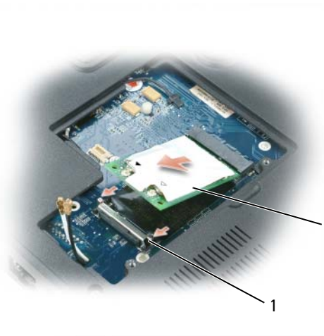
1 固定夾 2 迷你卡
