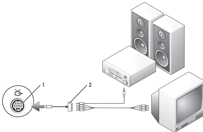
1 分離式影像電視輸出連接器 2 元件影像配接器
