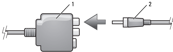
1 合成式影像配接器 2 S/PDIF 數位音效纜線
