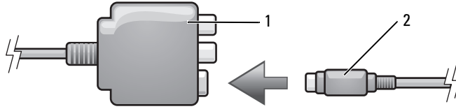
1 合成式影像配接器 2 S-video 纜線
