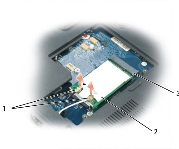
1 天線纜線 (2) 2 迷你卡 3 迷你卡連接器
